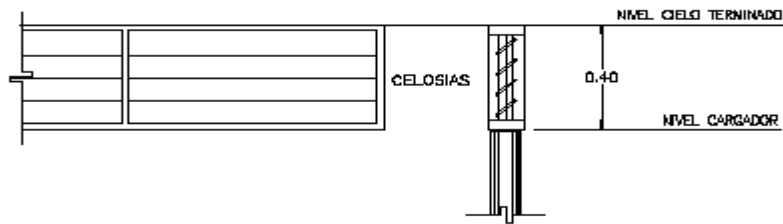
DETALLES DE VENTANERIA A CAMBIAR TIPO 3
