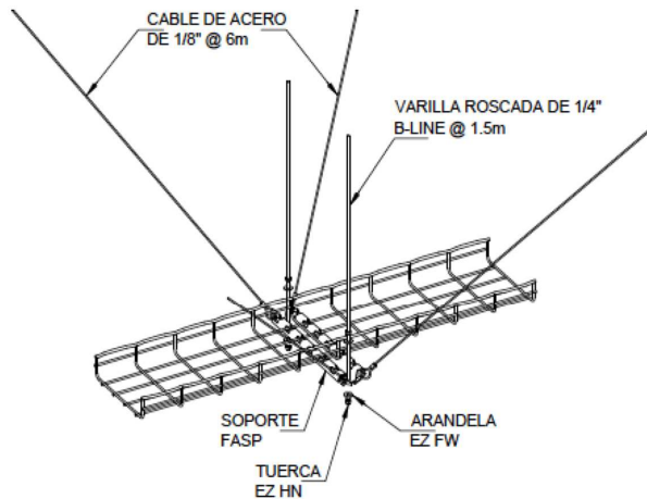
DETALLE SOPORTE ANTISISMICO PARA CANASTA SIN ESCALA
