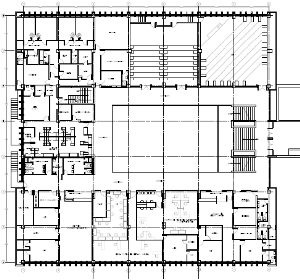
1º PISO TRIBUNALES DE SAN RAMON
