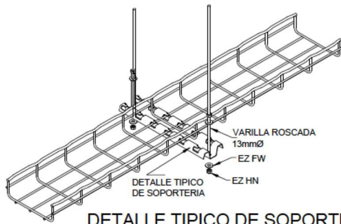
DETALLE TIPICO DE SOPORTERIA SIN ESCALA
