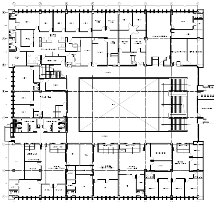
2° PISO TRIBUNALES DE SAN RAMÓN 1671,00 m2 (1629,00 elctricoo)
